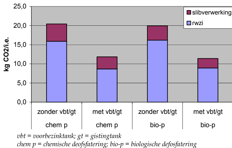
FIGUUR 4.1 KILOGRAM CO 2 /I.E. TEN GEVOLGE VAN PRIMAIR ENERGIEVERBRUIK VOOR VERSCHILLENDE TYPEN RWZI'S EN GEMIDDELDE SLIB-EINDVERWERKING
